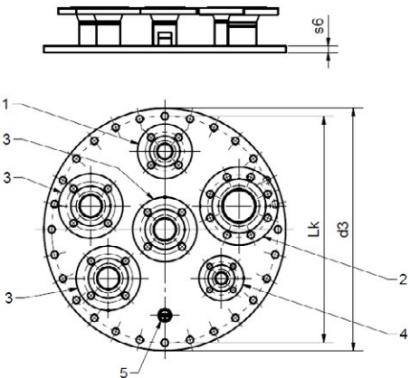
Domdeckel mit Flanschanschlüssen
