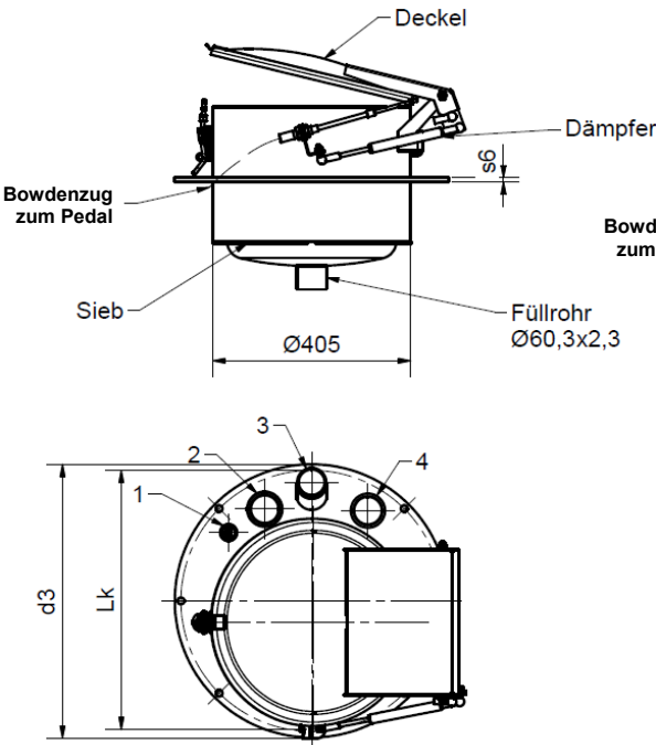
Domdeckel DN500 mit Einfülltrichter
